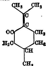
Pulegone.
